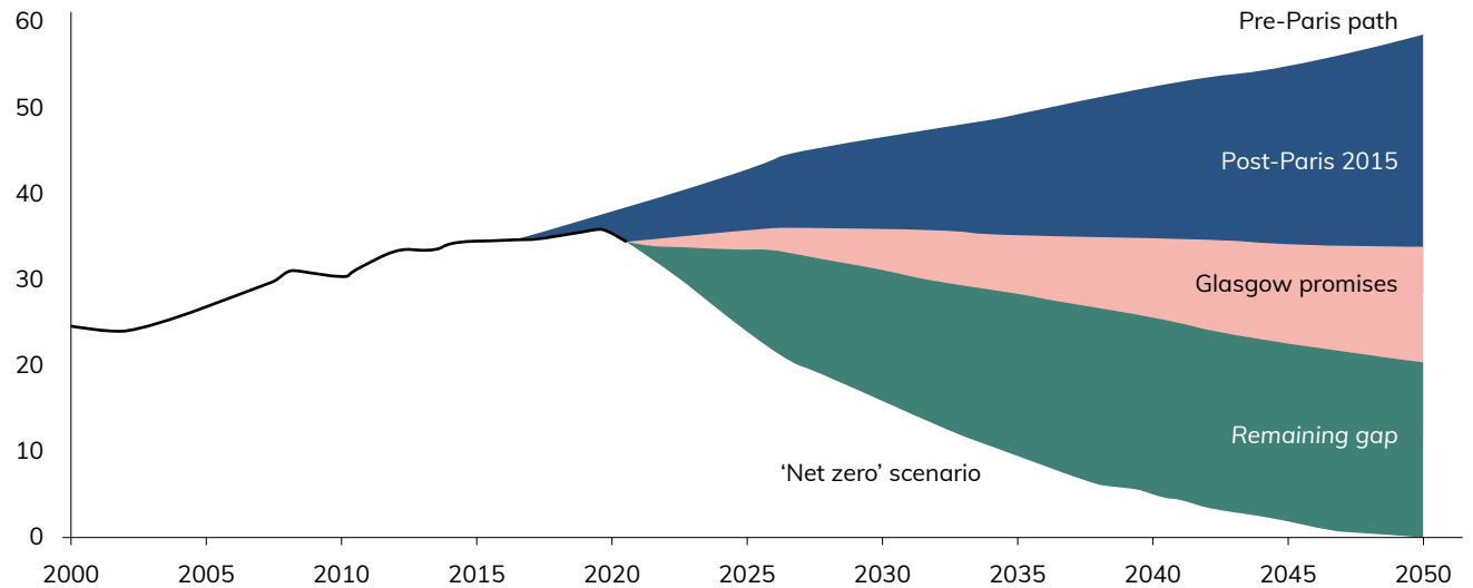
CO 2 EMISSIONS IN THE WORLD PER SCENARIO, 2000-2050
